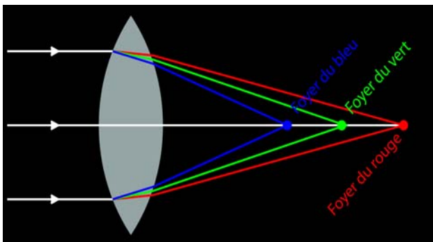
Fig.1. Chromatisme d'une lentille
