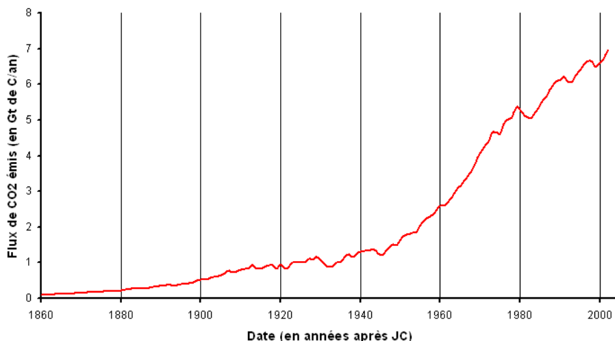
Flux d'émission de CO 2 liée à la combustion des carburants fossiles
