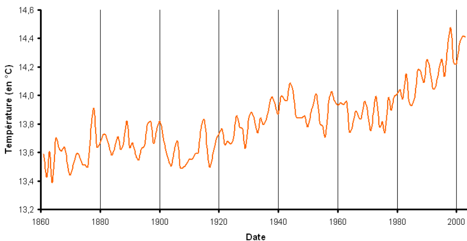
Moyennes annuelles des températures globales (Océans et continents)
