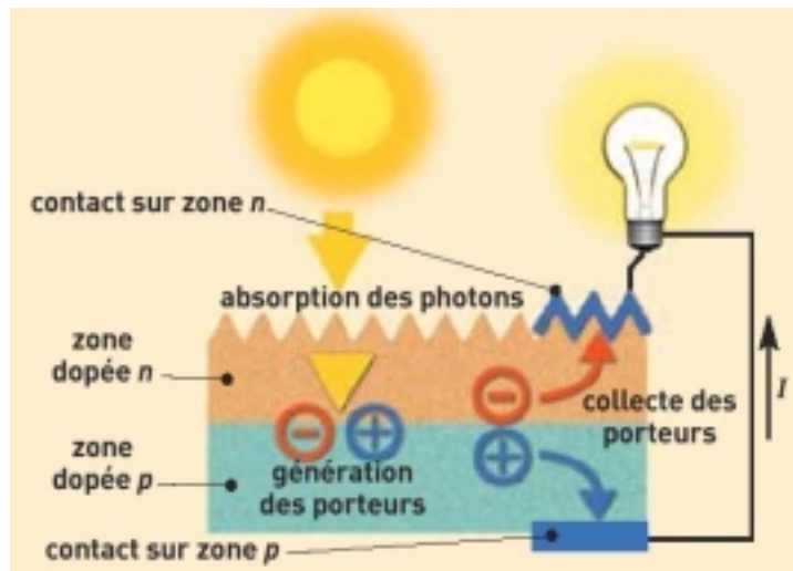
Principe de fonctionnement d'une cellule photovoltaïque. Source : http://www.cea.fr/fr/Publications/clefs50/encadred.pdf
