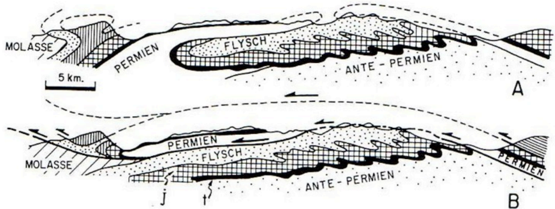
Fig. 11 - La structure des Alpes de Glaris (d'après Bailey 1935, modifié). a) l'hypothèse du double pli de Heim. b) l'hypothèse d'un charriage unique vers le nord de Bertrand.
